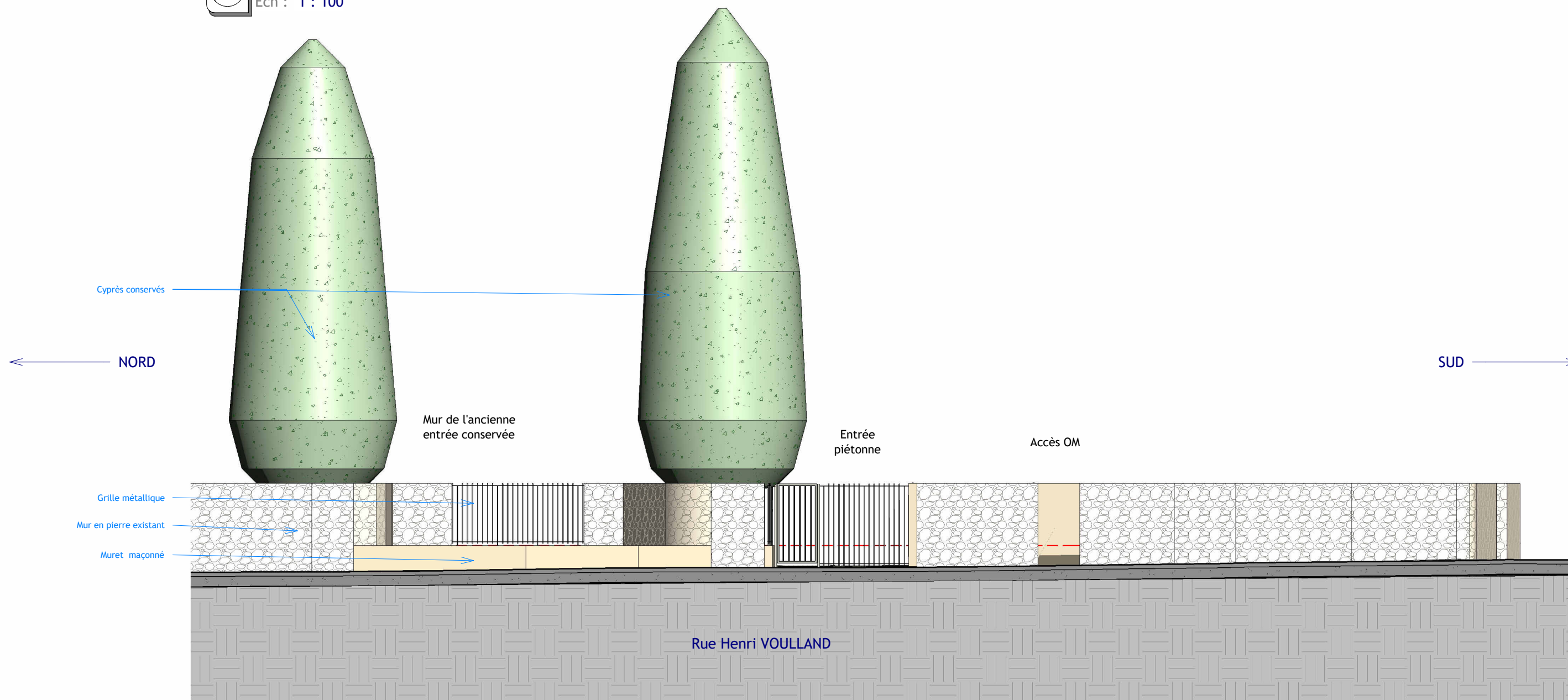
2 LIMITE RUE VOULLAND Ech : 1 : 100
