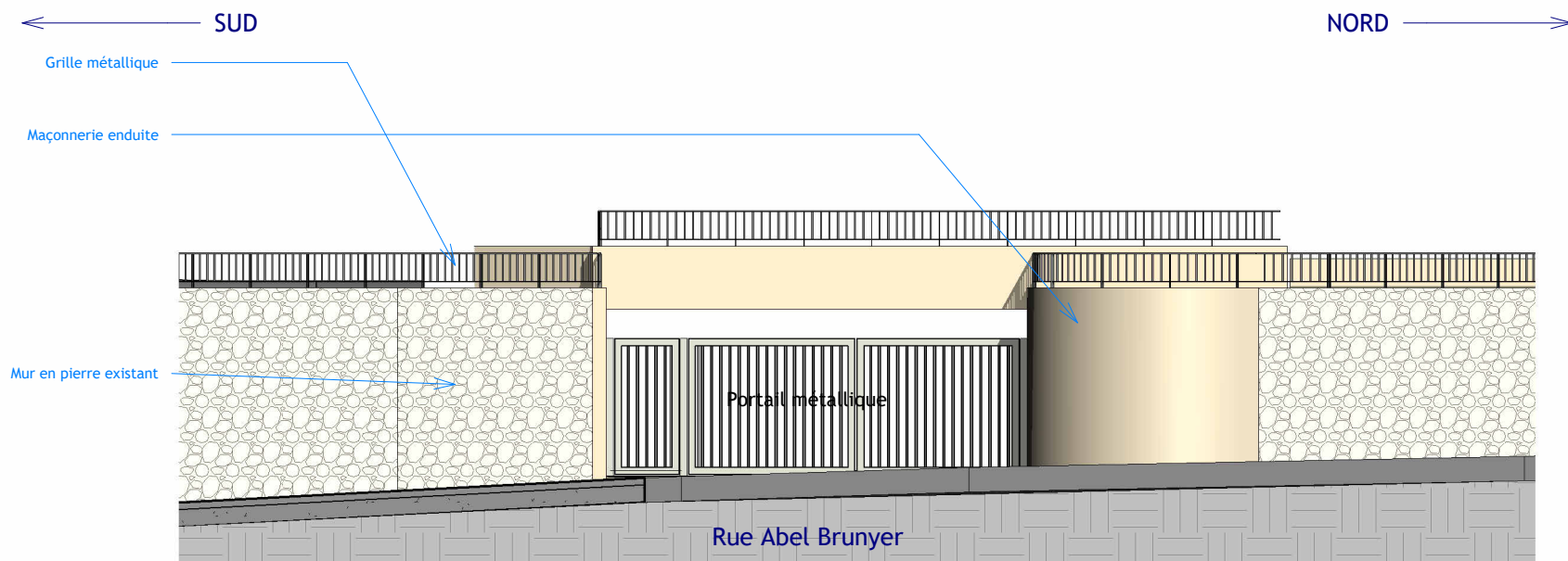
1 LIMITE R. BRUNYER Ech : 1 : 100
