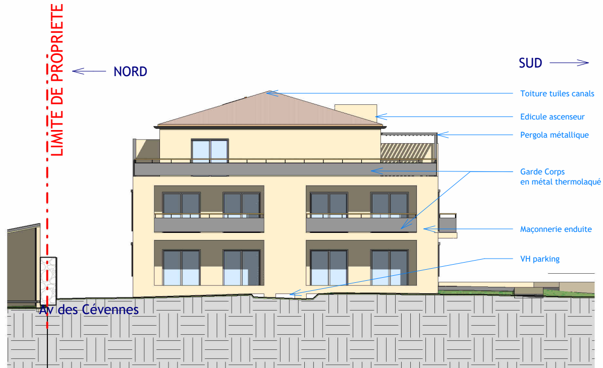
2 EL-OUEST-BAT-A Ech : 1 : 200
